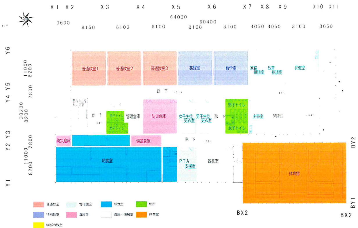
1階平面図
